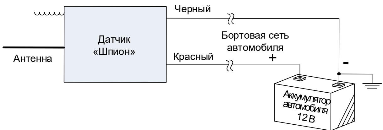
Рисунок Г.3 - Схема подключения Шпион
