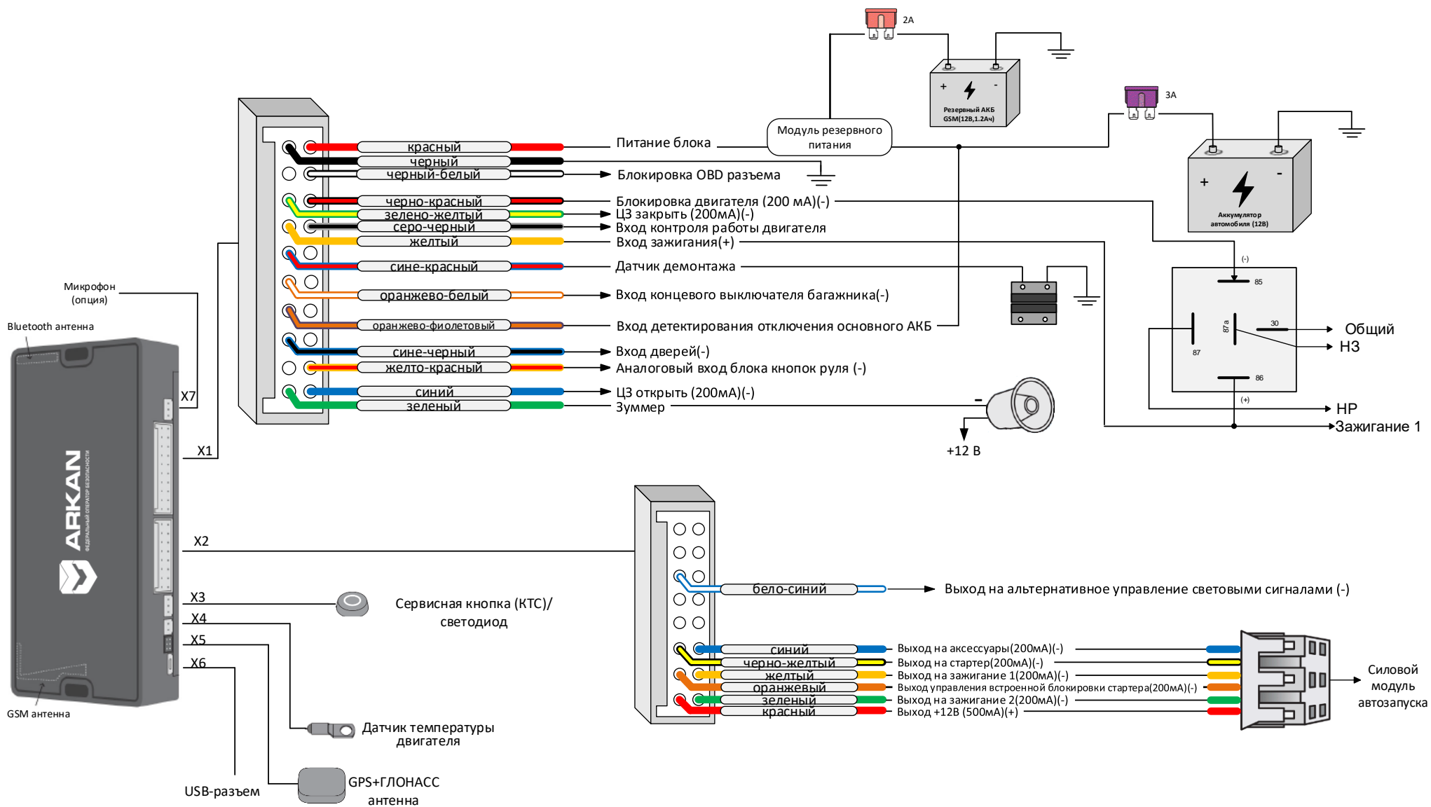
Рисунок А.2 – Схема аналогового подключения Комплекса (исп. Artset Pro, Artset Pro Spb комплектации «Smart») без CAN-модуля (Тип блокировки программируется через ARKAN Мастер)
