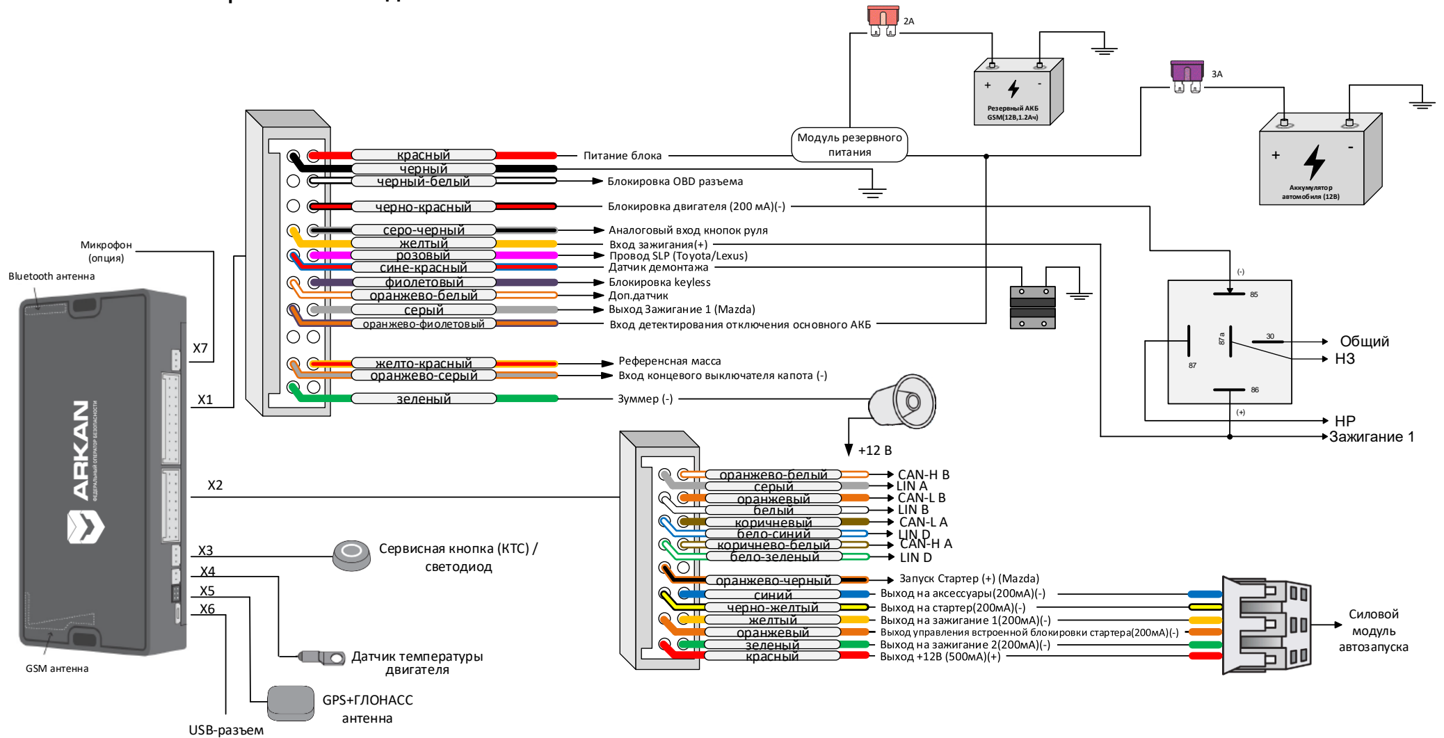
Рисунок А.1 – Схема подключения Комплекса со встроенным CAN-модулем (Тип блокировки программируется через ARKAN Мастер)
