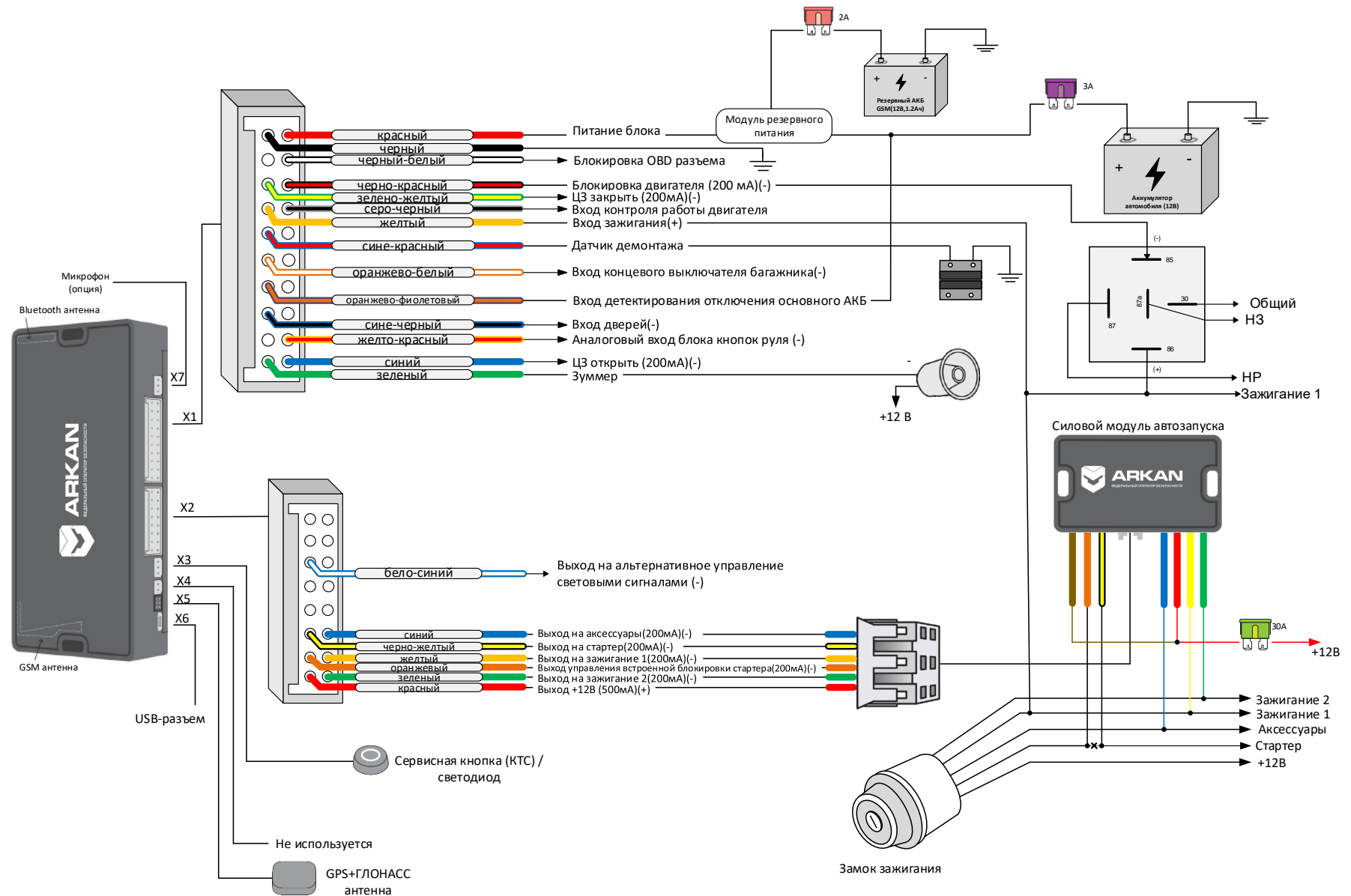
Рисунок А.3 – Схема аналогового подключения Комплекса (исп. Artset Pro, Artset Pro Spb комплектации «Smart A») без CAN-модуля (Тип блокировки программируется через ARKAN Мастер)
